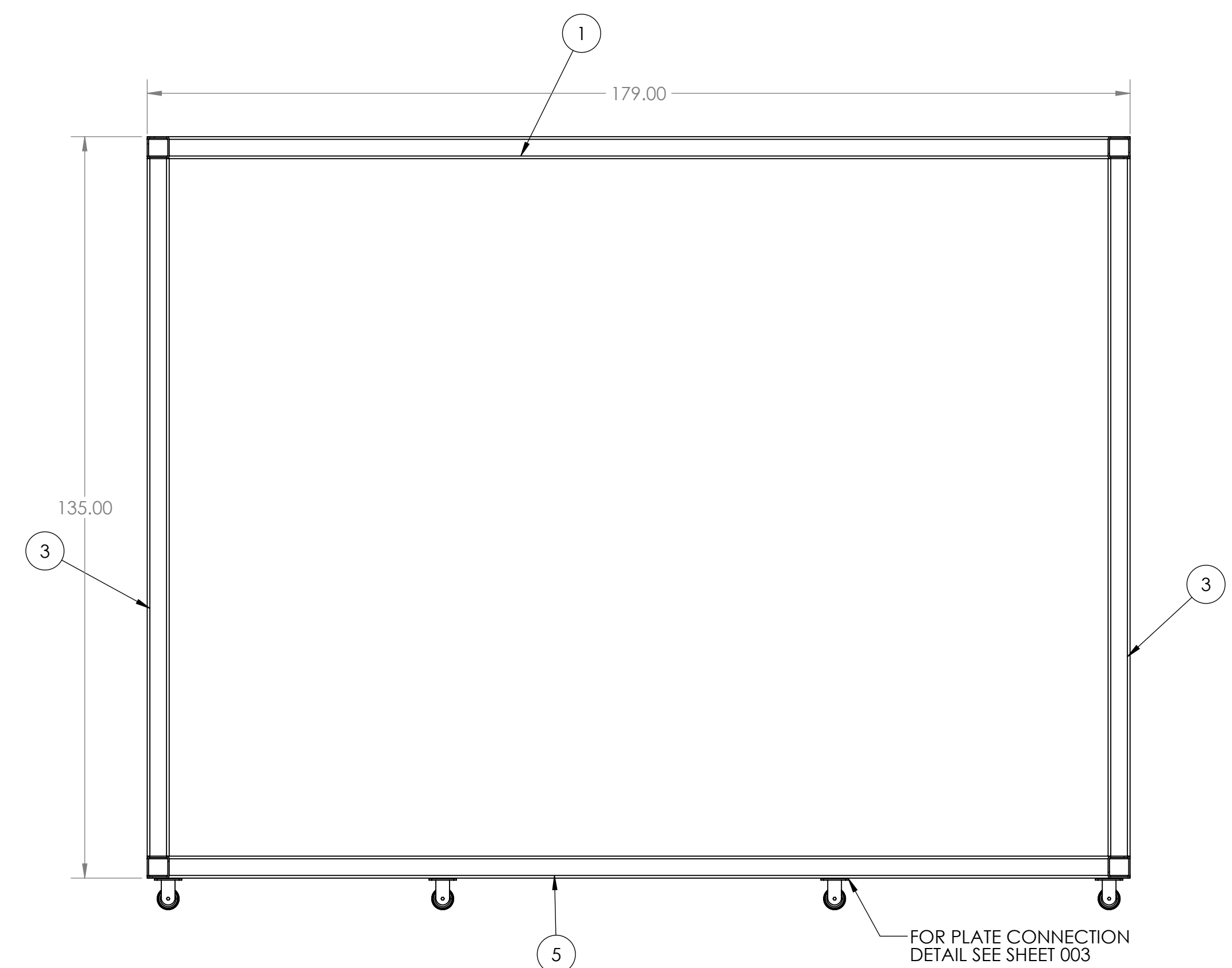
SECTION A-A SCALE 1:20
